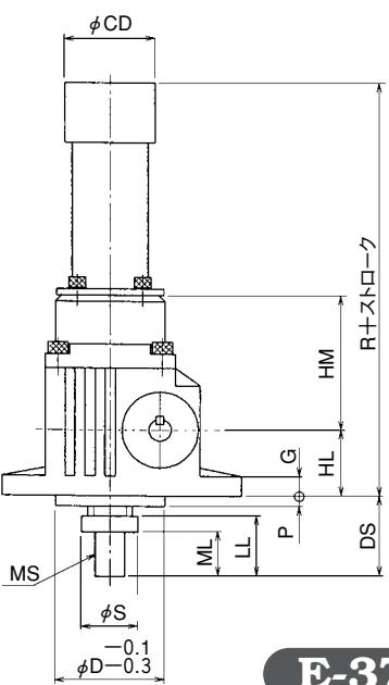
D (引上型)
