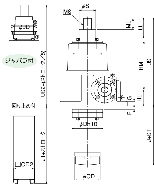
押上型
