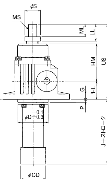
U (押し型)
