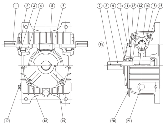
構造図W代表例です
