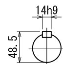
出力軸 (尺度1/4)
