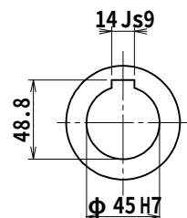
出力軸
