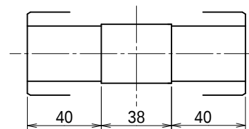
出力軸内部詳細 (尺度 1/2)
