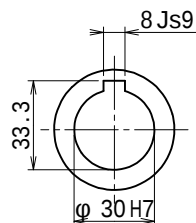
出力軸 (尺度 1/2)
