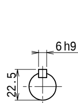
入力軸 (尺度 1/2)
