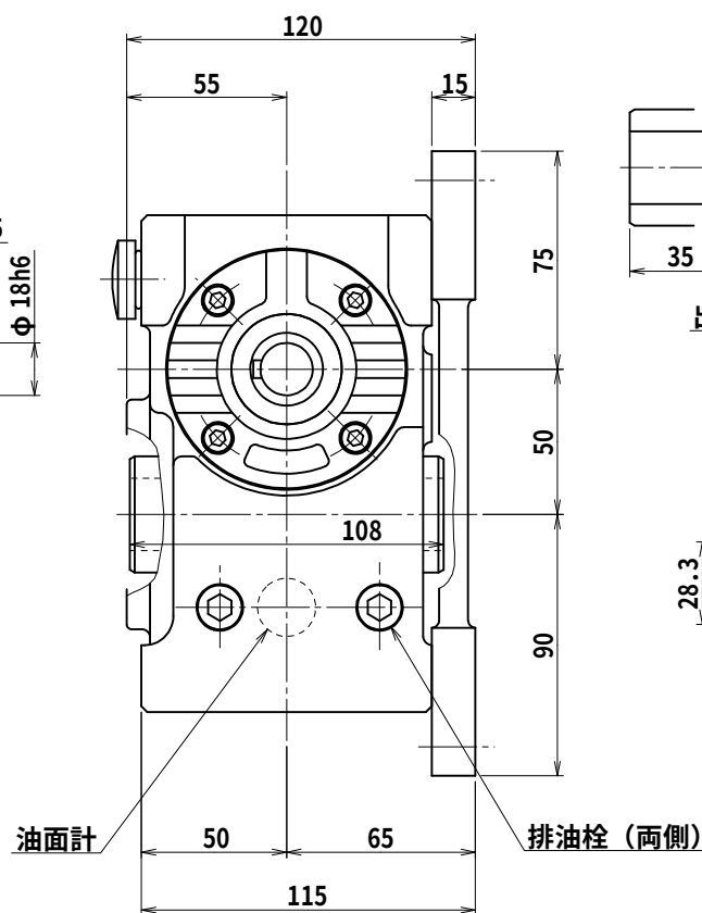
出力軸 (尺度 1/2)
