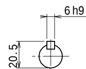
入力軸 (尺度 1/2)
