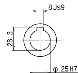
出力軸 (尺度 1/2)
