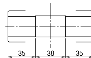
出力軸内部詳細 (尺度 1/2)
