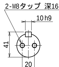
出力軸 (尺度 1/2.5)
