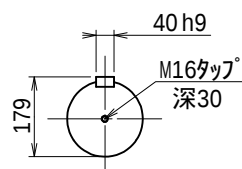
出力軸
