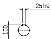
入力軸
