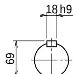
出力軸 (S=1/5)
