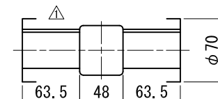
出力軸中空軸詳細 (尺度1/4)
