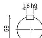
出力軸 (尺度 1/3)
