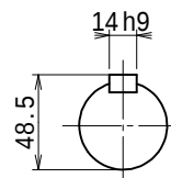
出力軸 (尺度 1/3)
