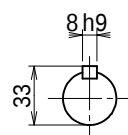
入力軸 (尺度 1/3)
