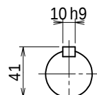
出力軸 (尺度 1/3)
