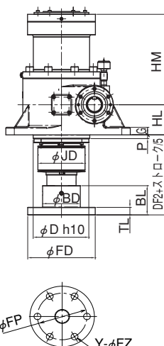
フランジエンドの場合
