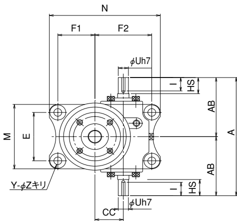
入力軸詳細
