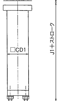
回り止め付
