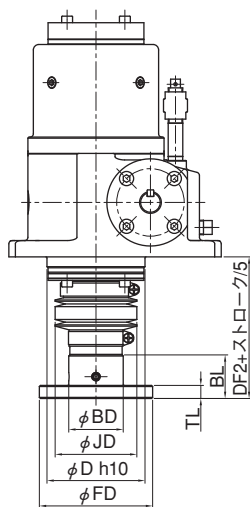
フランジエンドの場合
