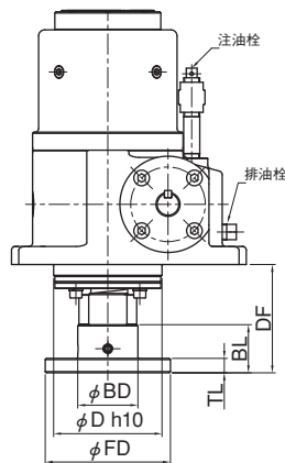
フランジエンドの場合
