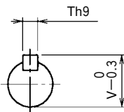
入力軸詳細
