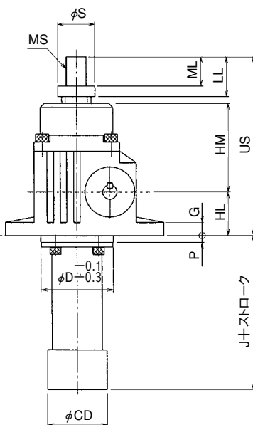
U(押上型)
