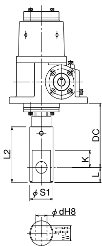
クレビスエンドの場合
