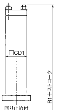
回り止め付
