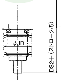
ジャバラ付
