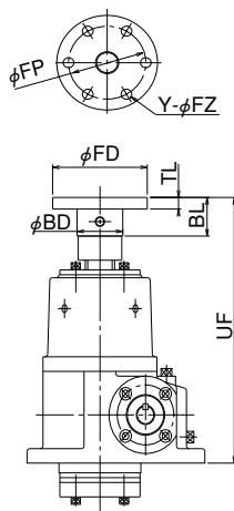
フランジエンドの場合
