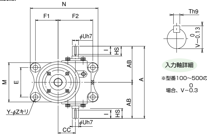
〈平面図〉
