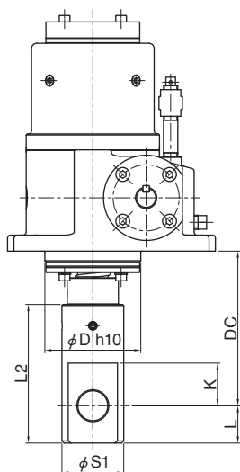
クレビスエンドの場合
