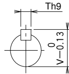
入力軸詳細
