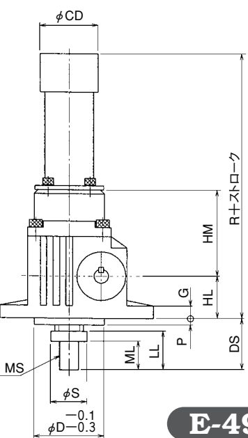
D(引上型)
