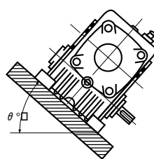
5 傾斜取付
