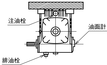
2 側面取付
