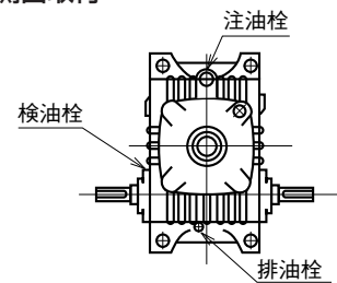
4 側面取付
