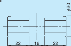
出力軸内部詳細 (S=1/1)
