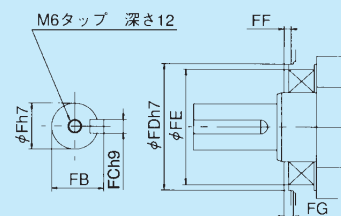
出力軸詳細
