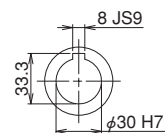
出力軸
