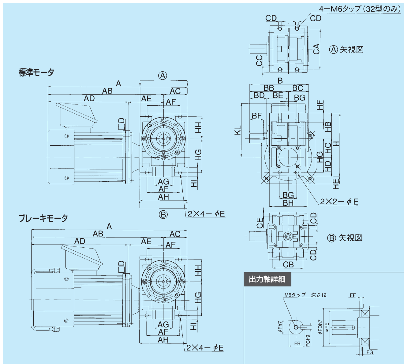
MA32・40 モータ付寸法
