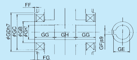
出力軸詳細
