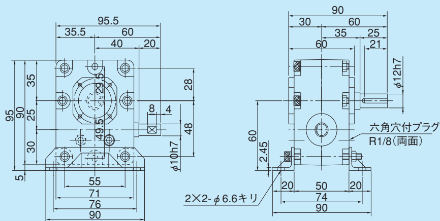
中実軸詳細図
