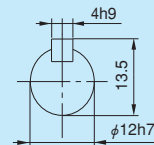
出力軸部詳細 (S=1/1)
