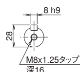
出力軸
