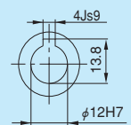
出力軸部詳細 (S=1/1)
